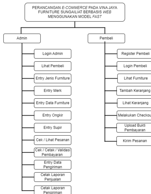
Gambar 3. Struktur Tampilan Layar
