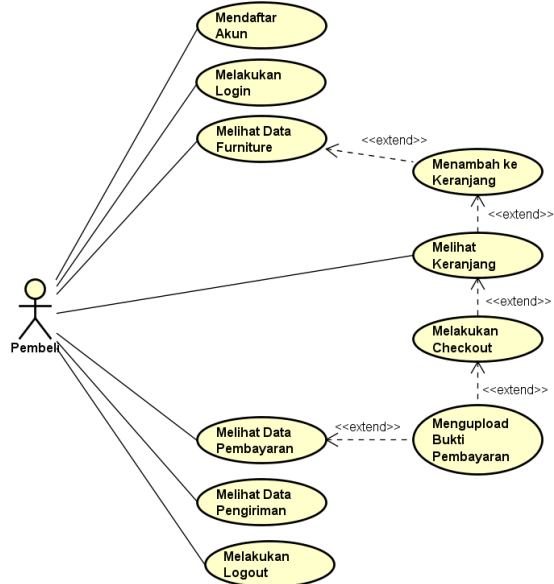
Gambar 5. Use case diagram pembeli
